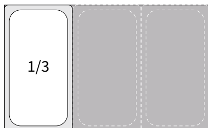
GN 1/3 rozměr 325 x 176 mm
