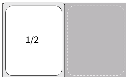
GN 1/2 rozměr 325 x 265 mm
